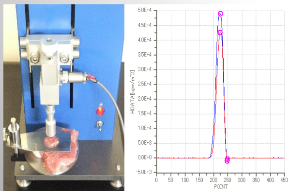
TENSIPRESSER † TTP-50BX2-2006 (タケトモ電機製)
